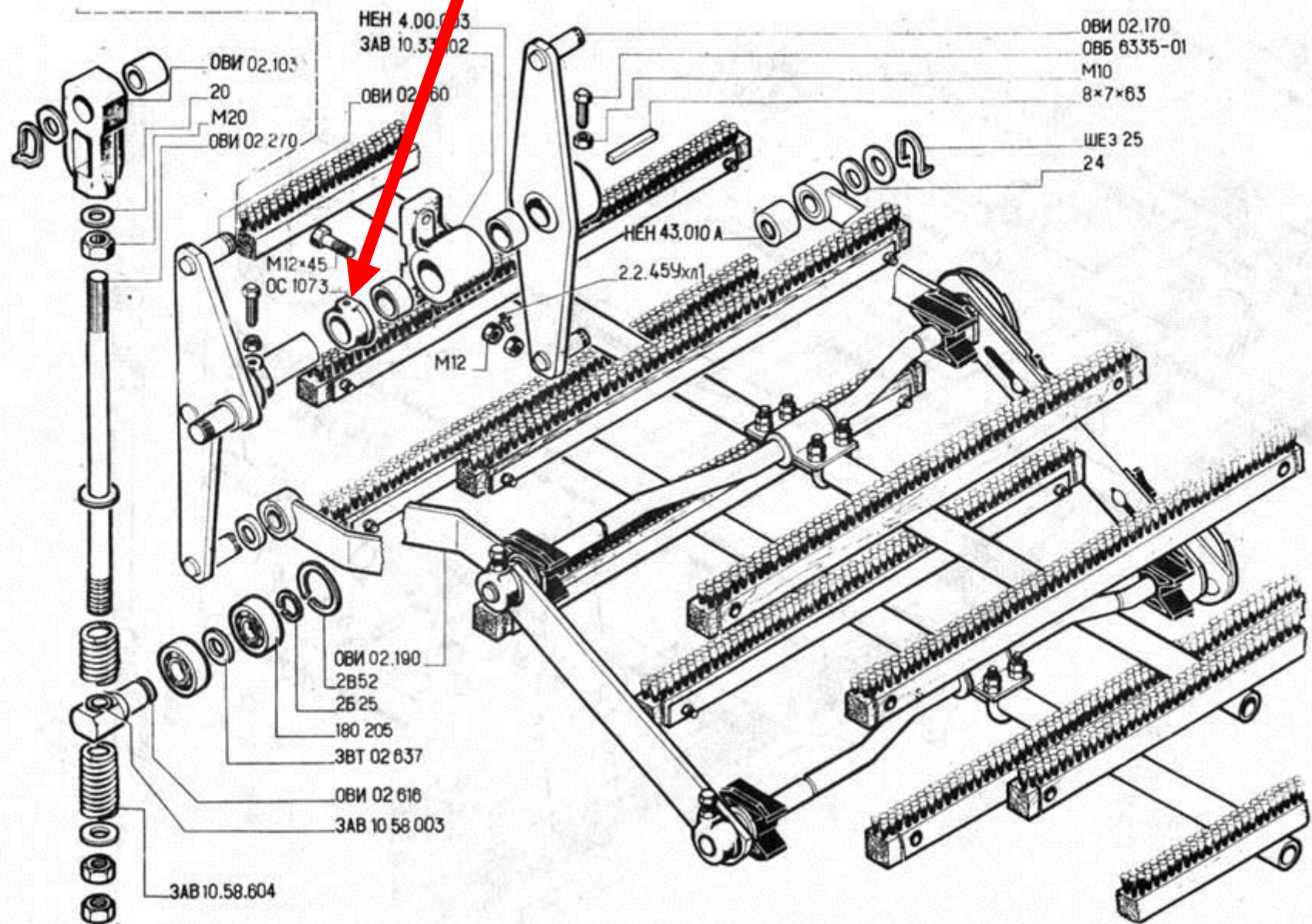
Рис. 12. Механизм очистки решет ОБИ 02.150.
